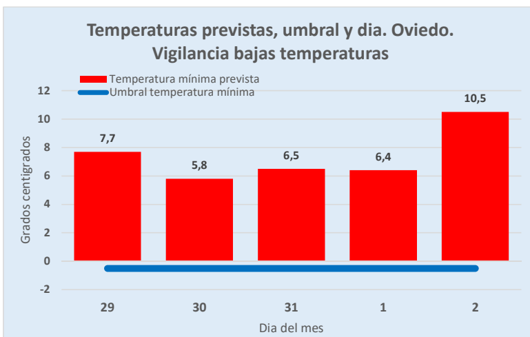
Predicción de AEMET a día de hoy. Comunicada por Ministerio de Sanidad.
